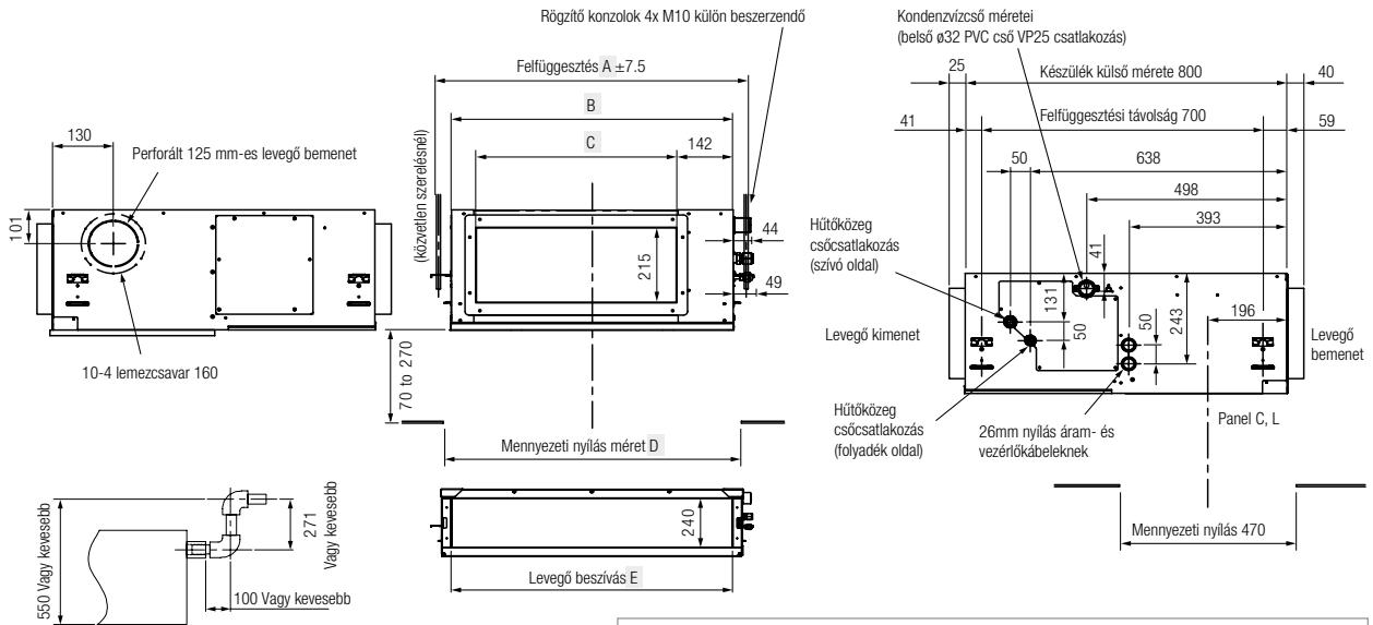
Kondenzvízcső méretei
