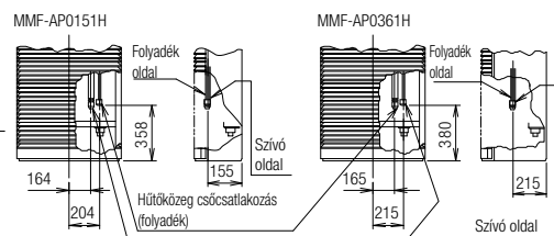
Hűtőközeg csatlakozások
